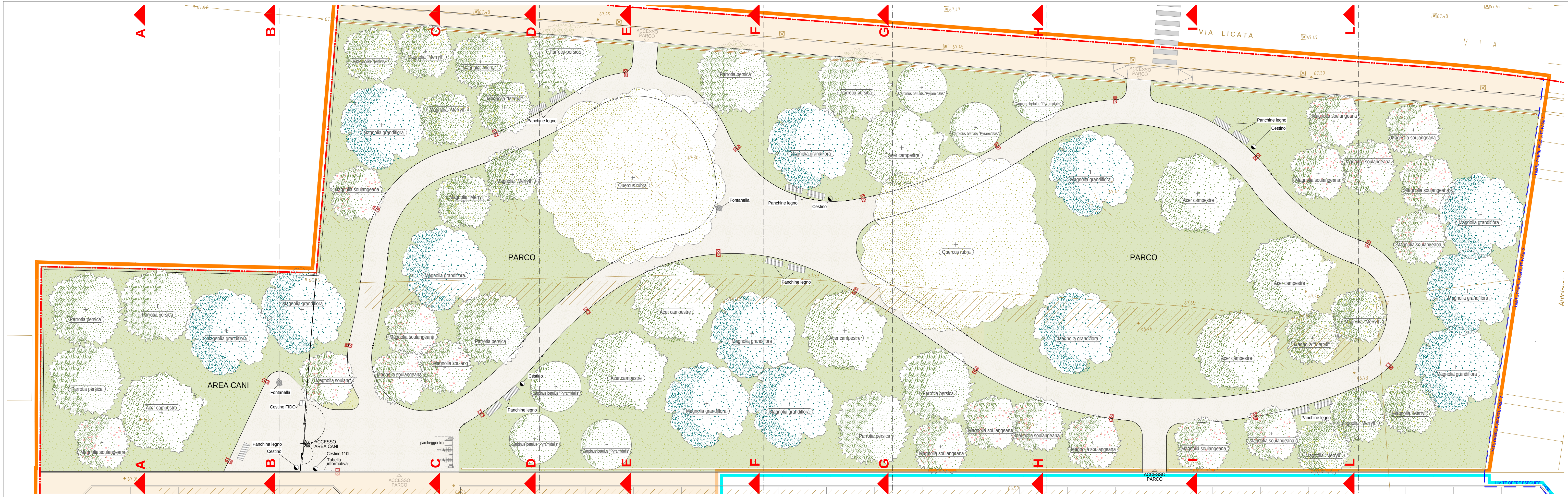
Planimetria generale 1:200
